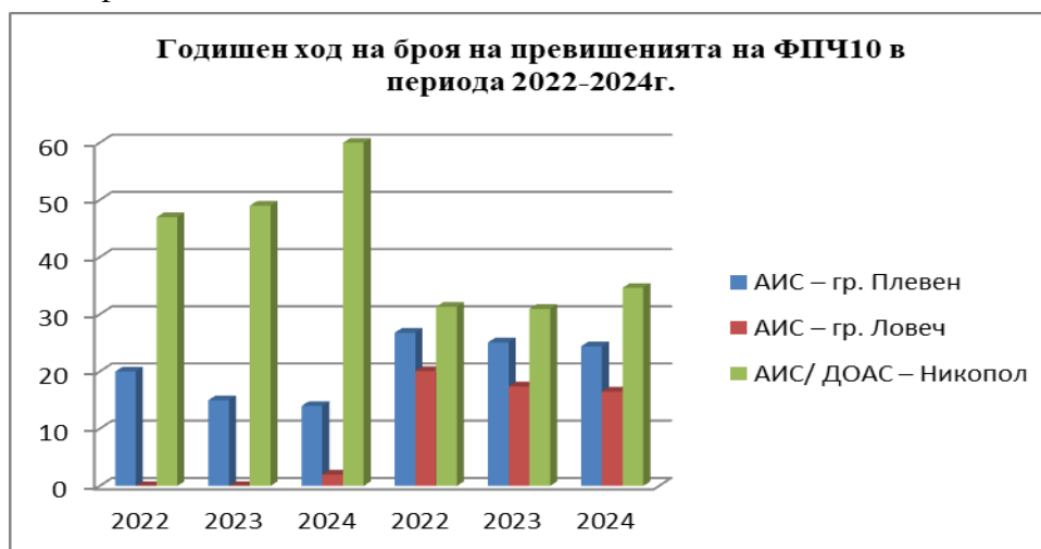
Фиг. 1. Брой денонощия с превишена СДН на ФПЧ 10 за периода 2022 – 2024 г.
