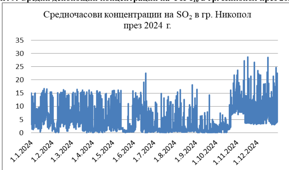
Фиг. 10. Средночасови концентрации на \text{SO}_2 в гр. Никопол през 2024 г.
