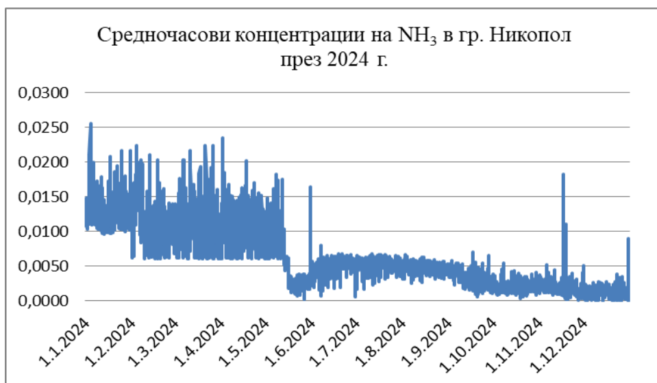
Фиг. 15. Средночасови концентрации на NH_3 в гр. Никопол през 2024 г.
