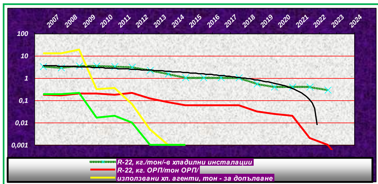
Фиг. 19. Употребата на фреон R-22 за периода 2007-2024 г. от оператори на хладилни инсталации и ремонтна дейност
