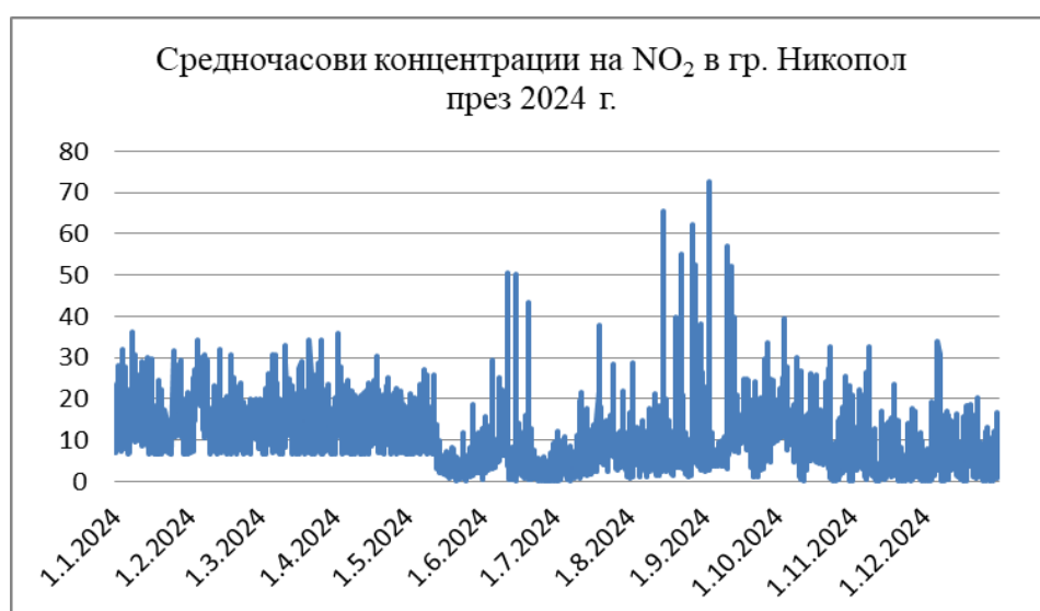
Фиг. 12. Средночасови концентрации на \text{NO}_2 в гр. Никопол през 2024 г.
