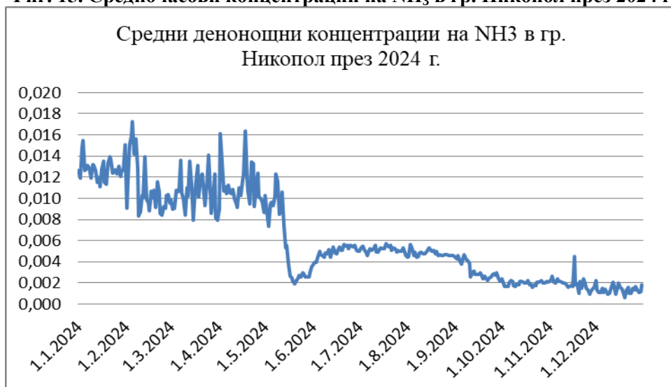
Фиг. 16. Средни денонощни концентрации на NH_3 в гр. Никопол през 2024 г.
