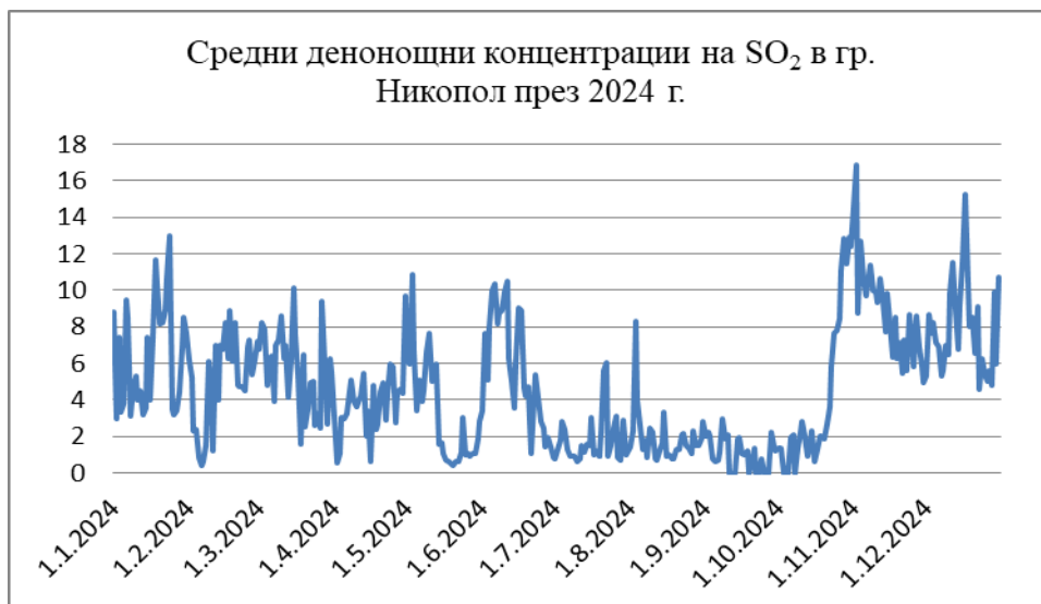
Фиг. 11. Средни денонощни концентрации на \text{SO}_2 в гр. Никопол през 2024 г.
