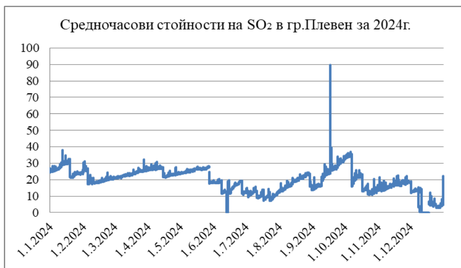
Фиг. 3. Средночасови концентрации на SO 2 в гр. Плевен през 2024г.
