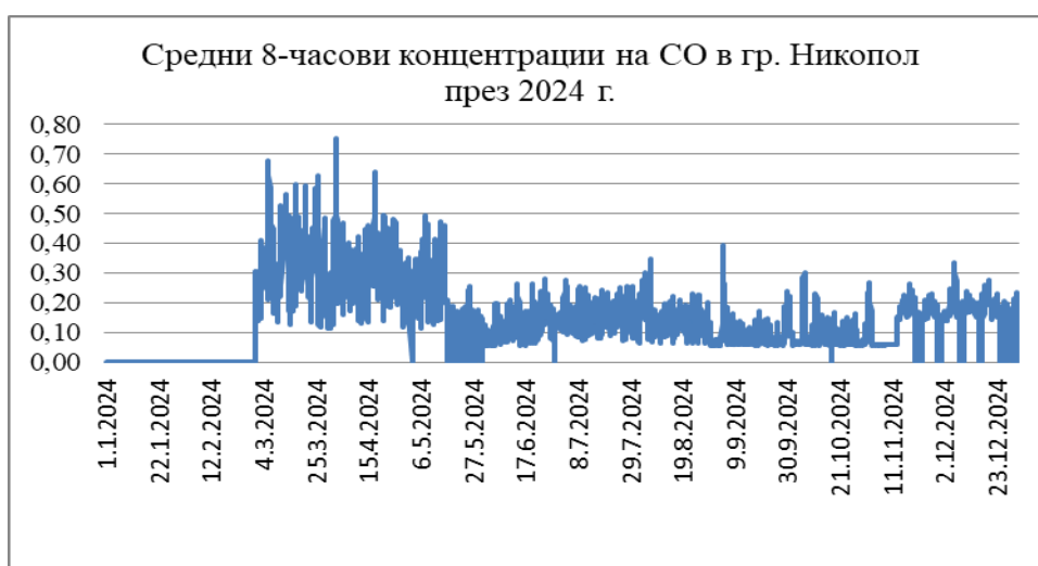
Фиг. 13. Средни 8-часови концентрации на \text{CO} в гр. Никопол през 2024 г.
