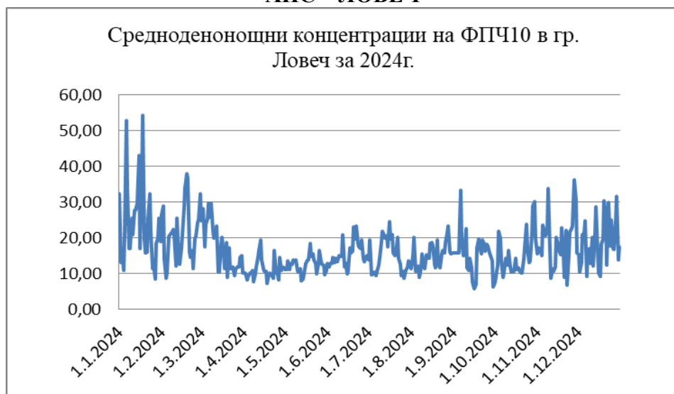
Фиг. 8. Средни денонощни концентрации на \text{ФПЧ}_{10} в гр. Ловеч през 2024г.
