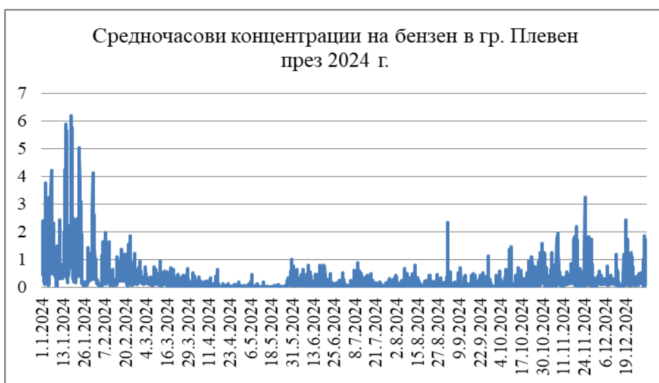
Фиг. 7. Средночасови концентрации на бензен в гр. Плевен през 2024г.
