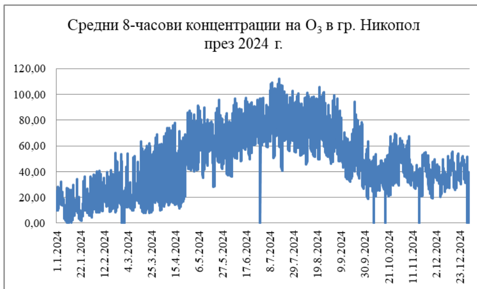
Фиг. 14. Средни 8-часови концентрации на O_3 в гр. Никопол през 2024 г.
